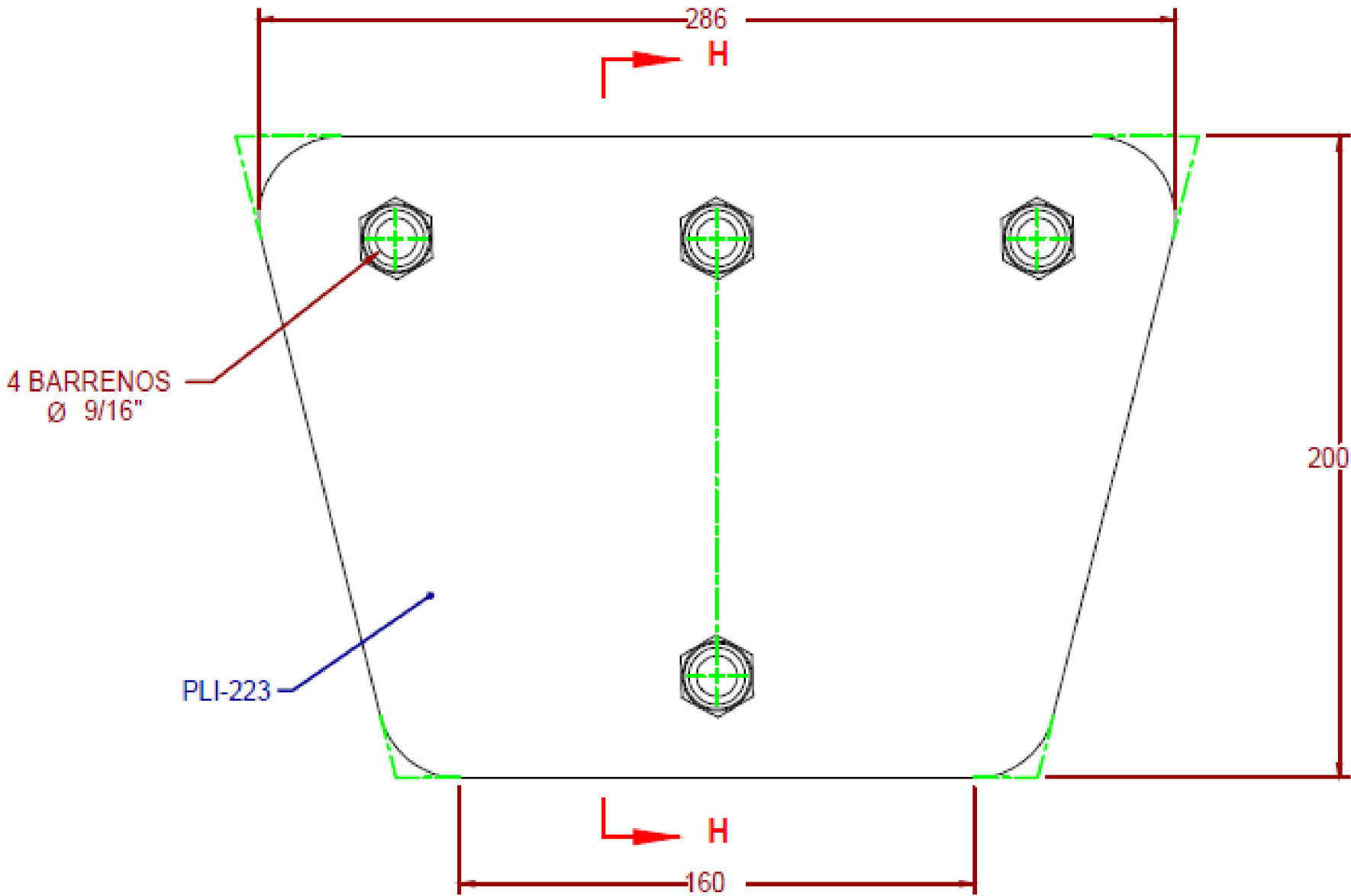
DETALLE DE ARMADO PLACAS IGUALADORAS 20-20-30
