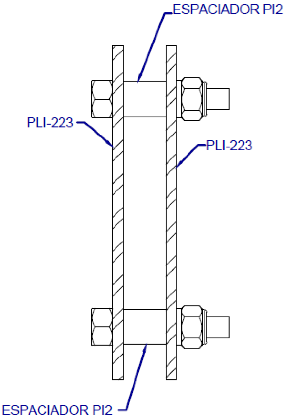
SECCIÓN H-H ESCALA 1:1.5
