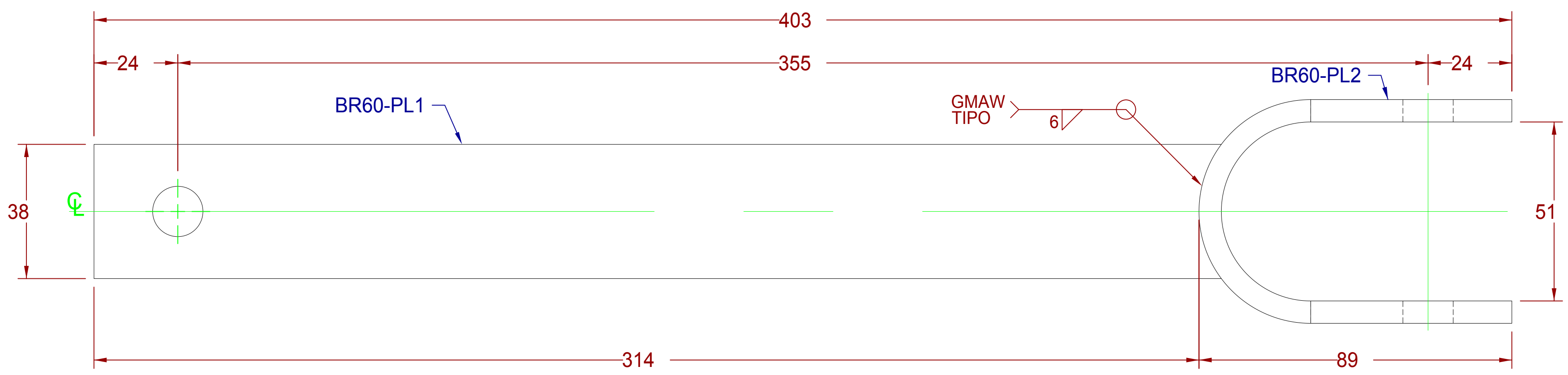
SECCIÓN A-A ESCALA 1:1
