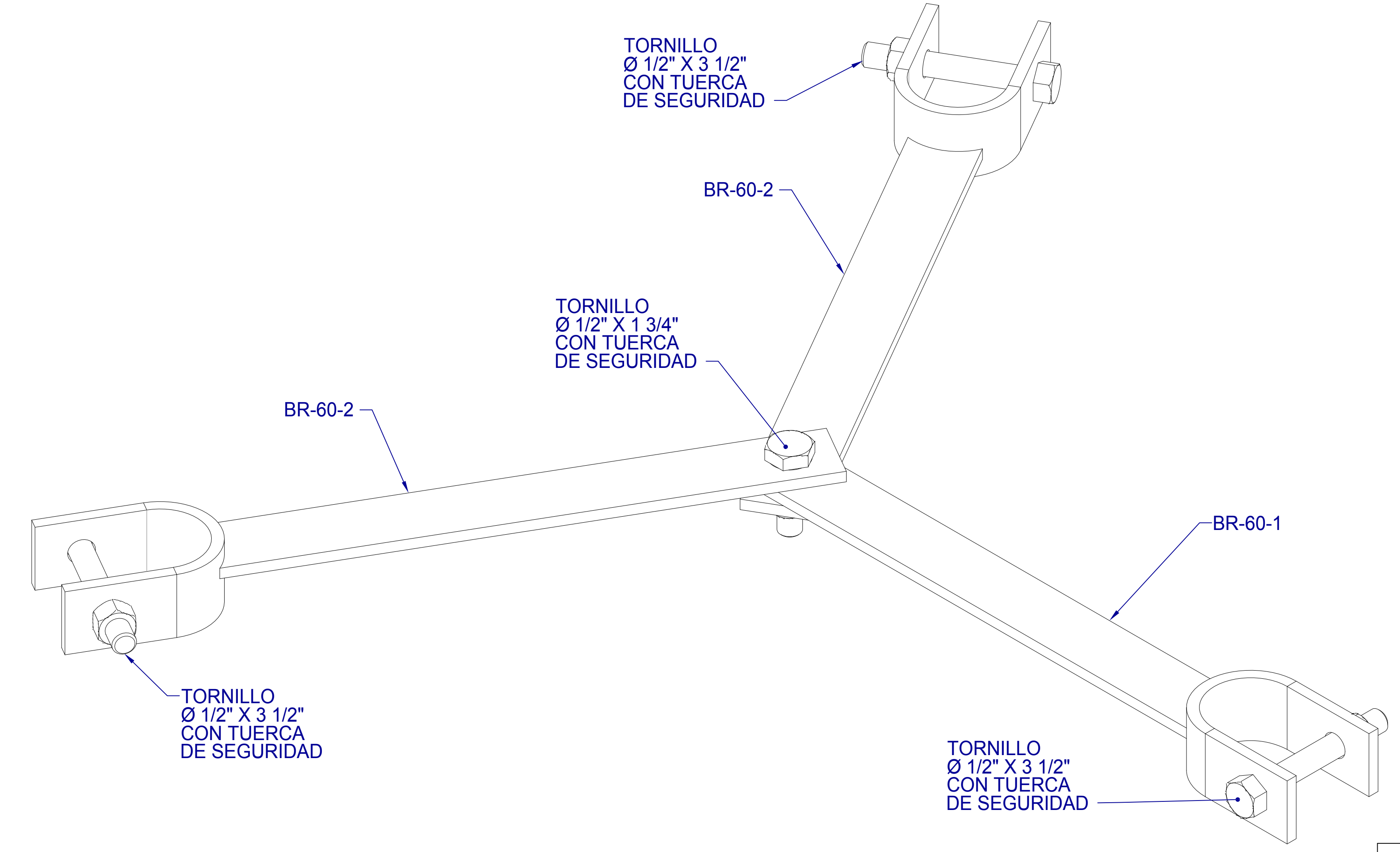
VISTA ISOMÉTRICA ENSAMBLAJE BRIDA 60
