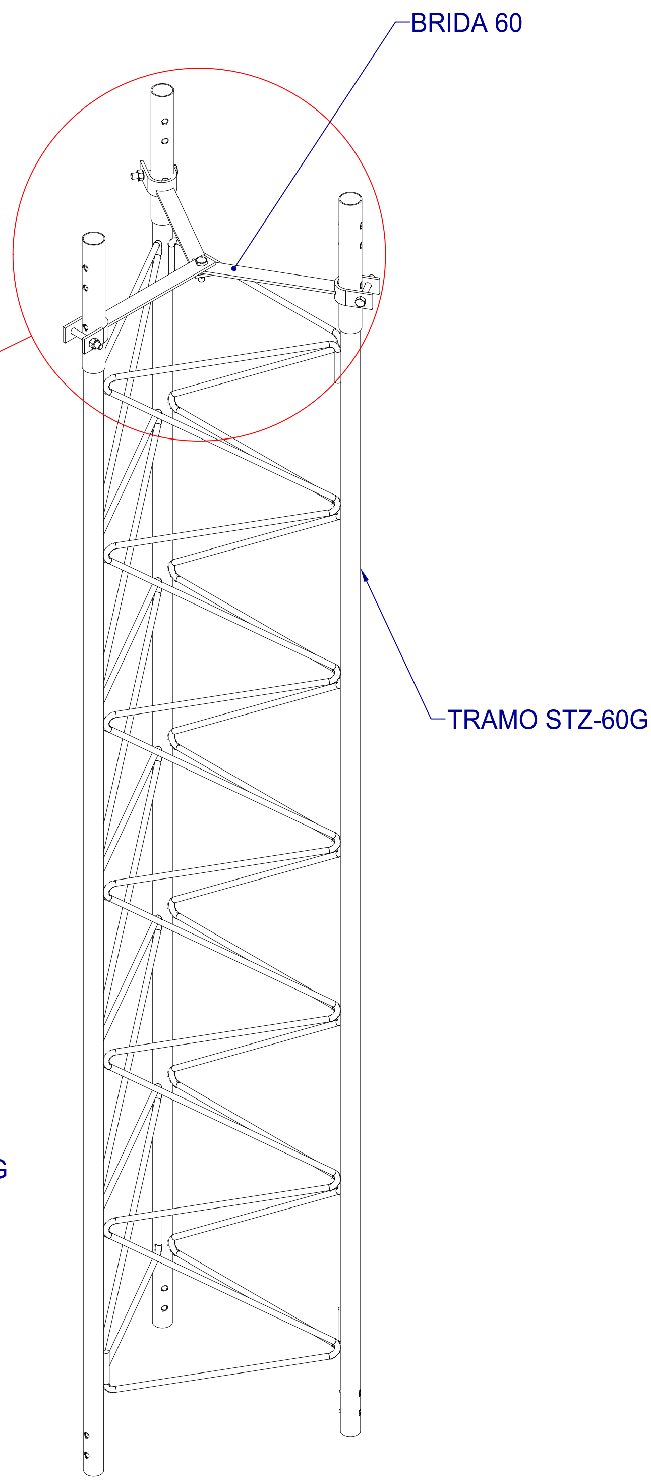
VISTA ISOMÉTRICA ENSAMBLAJE BRIDA 60 CON TRAMO STZ-60G
