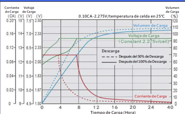
Curva característica de carga en flotante (25°C/77°F)
