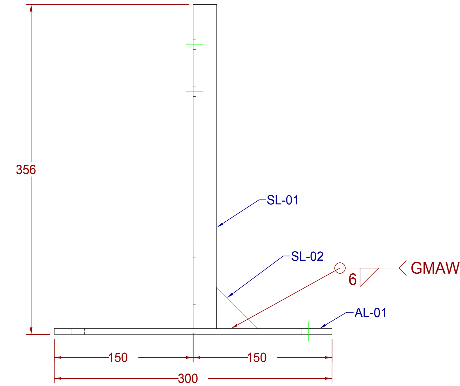
SECCIÓN U-U ESCALA 1 : 2.5
