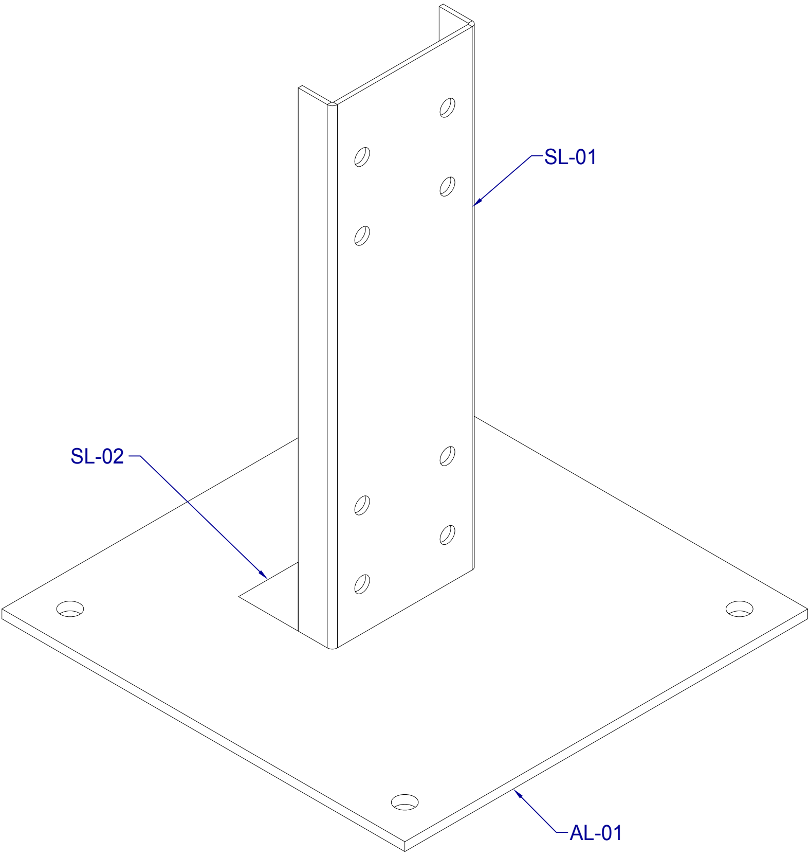
VISTA ISOMÉTRICA SLMBA4G BASE RECTA PARA MÁSTIL
