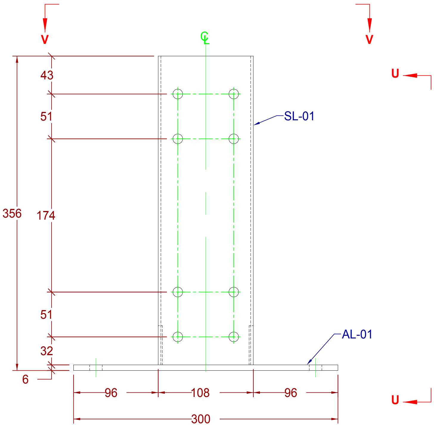
VISTA ELEVACIÓN SLMBA4G BASE RECTA PARA MÁSTIL
