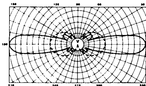
E-PLANE
